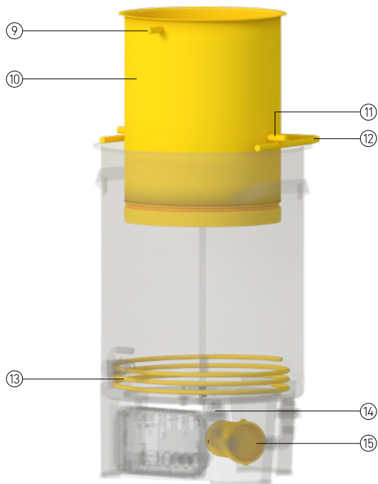
Braumeister PLUS 50 Liter während des Brauvorgangs beim Abläutern
